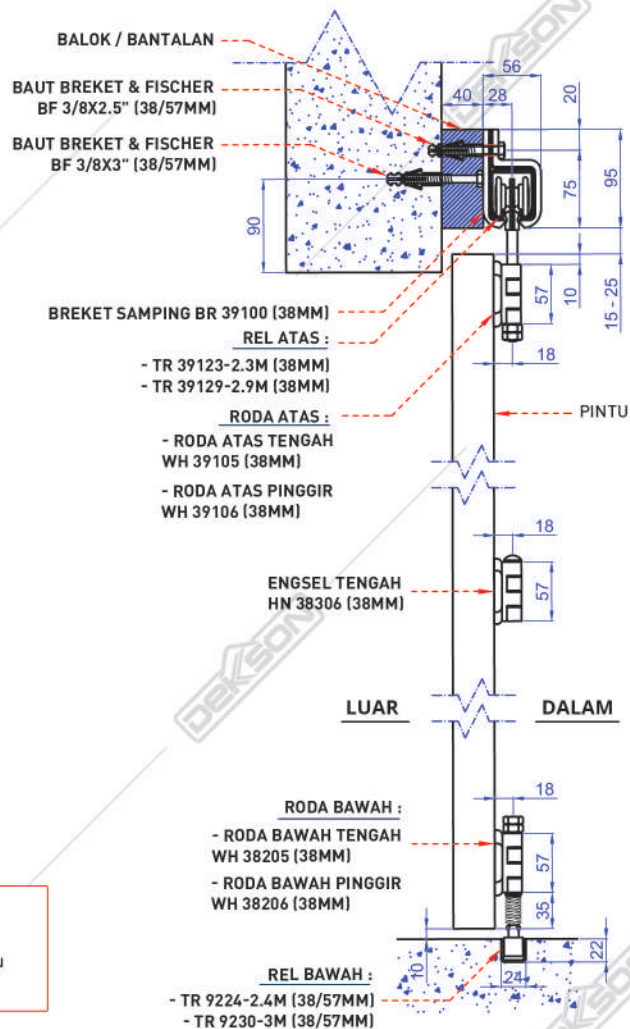
Gambar Potongan
