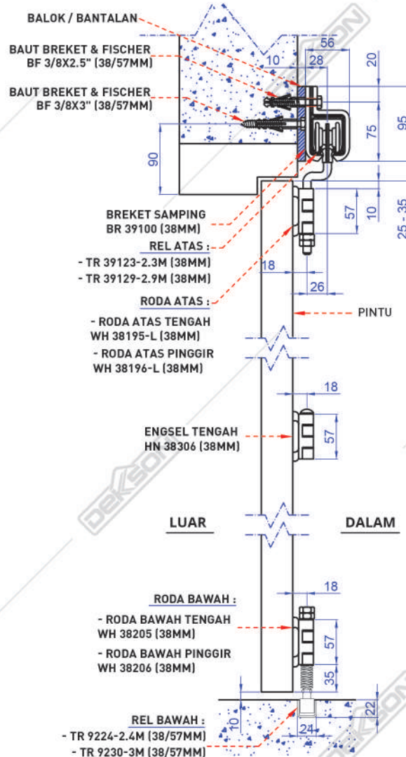
Gambar Potongan
