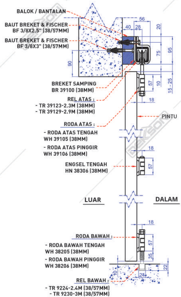
Gambar Potongan
