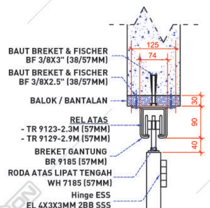
Gambar Potongan
