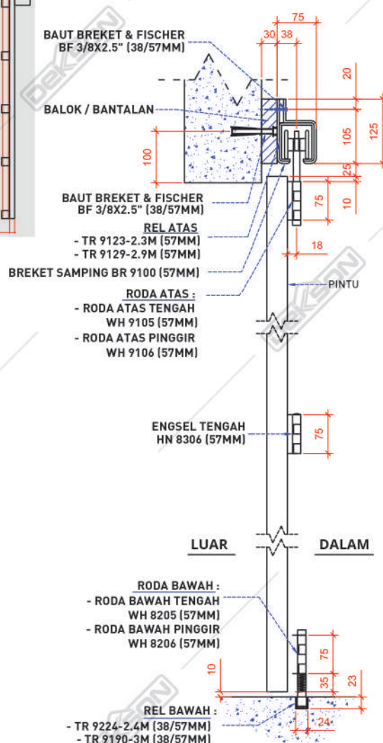
Gambar Potongan
