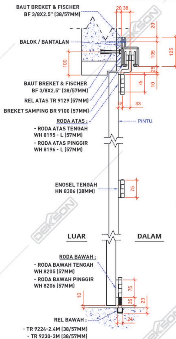
Gambar Potongan
