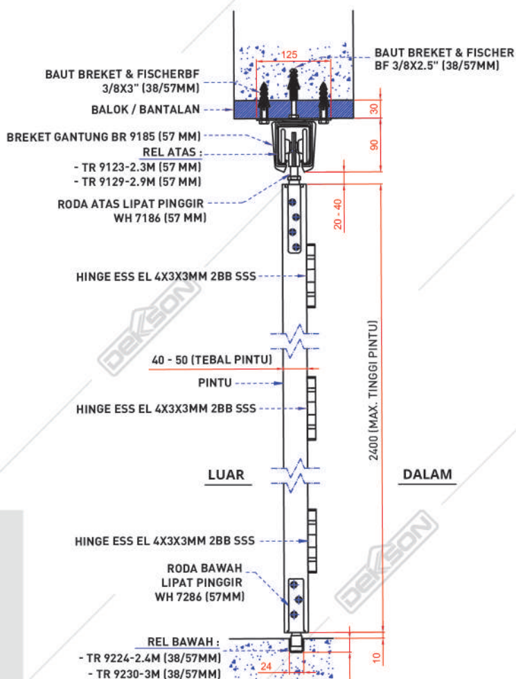
Gambar Potongan
